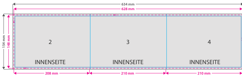
Falzbeispiel
